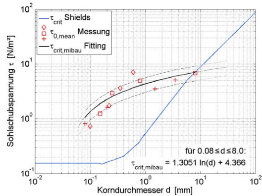
Ergebnisdiagramm der Versuchsserien zur Lagestabilität
